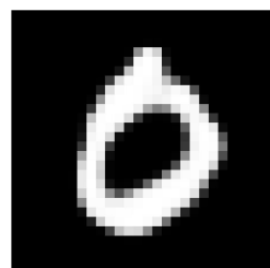
CAE
